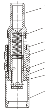
Fangvorrichtung pumpbar
