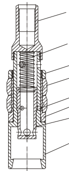
Fangvorrichtung pumpbar
