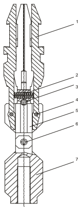
Klinkenkopf
