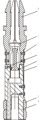
Klinkenkopf pumpbar
